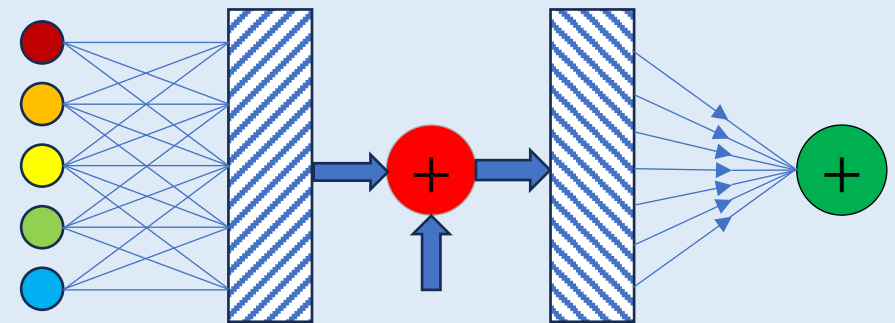
深層学習と繰り込み群
